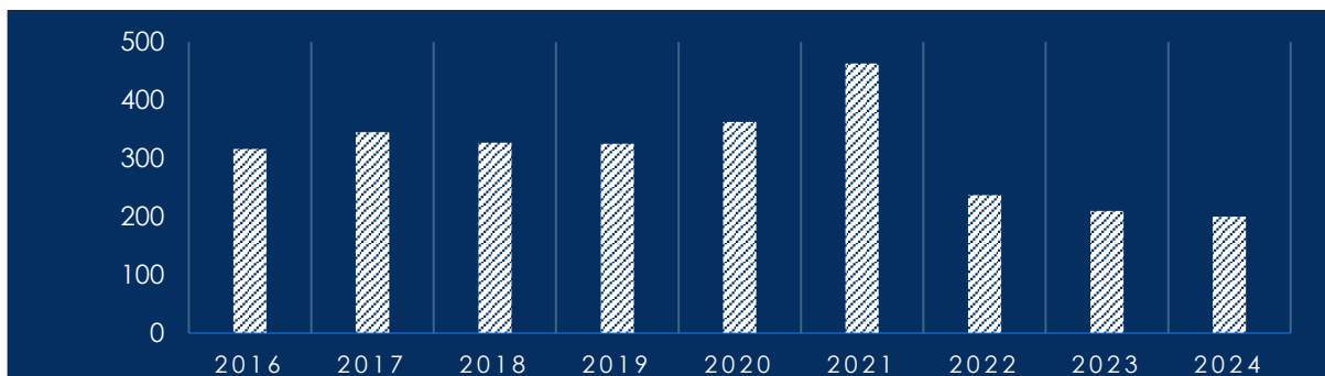
Рис. 2.25 Динаміка споживання електроенергії на вуличне освітлення, МВт*год
