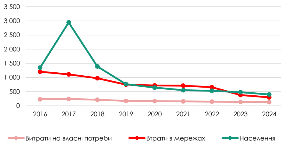
Рис. 2.30. Виробництво, втрати та споживання теплової енергії, Гкал
