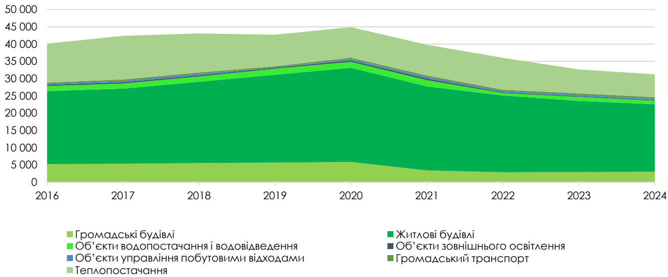
Рис. 2.37 Зведений енергетичний баланс за категоріями кінцевих споживачів за 2016-2024 роки
