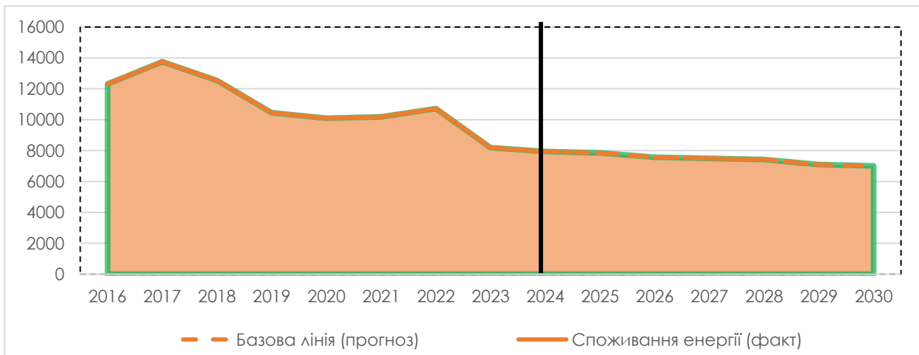
Рис 3.9 Фактичне та прогнозне споживання енергії у секторі теплопостачання.
