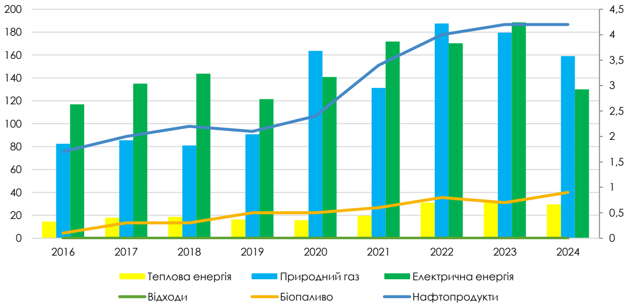
Рис 2.41 Зведений вартісний баланс за видами енергії, млн грн.
