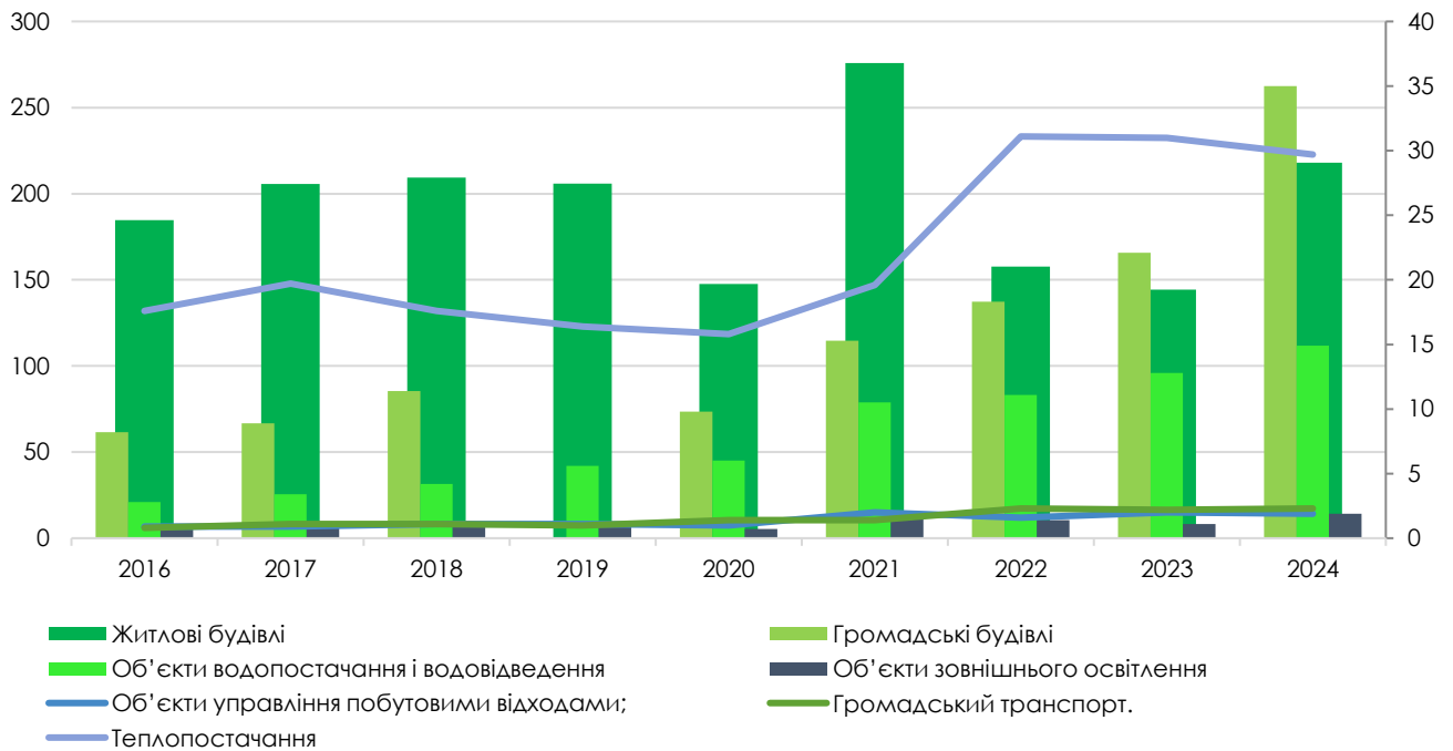
Рис 2.40 Зведений вартісний баланс за категоріями кінцевих споживачів, млн. грн.
